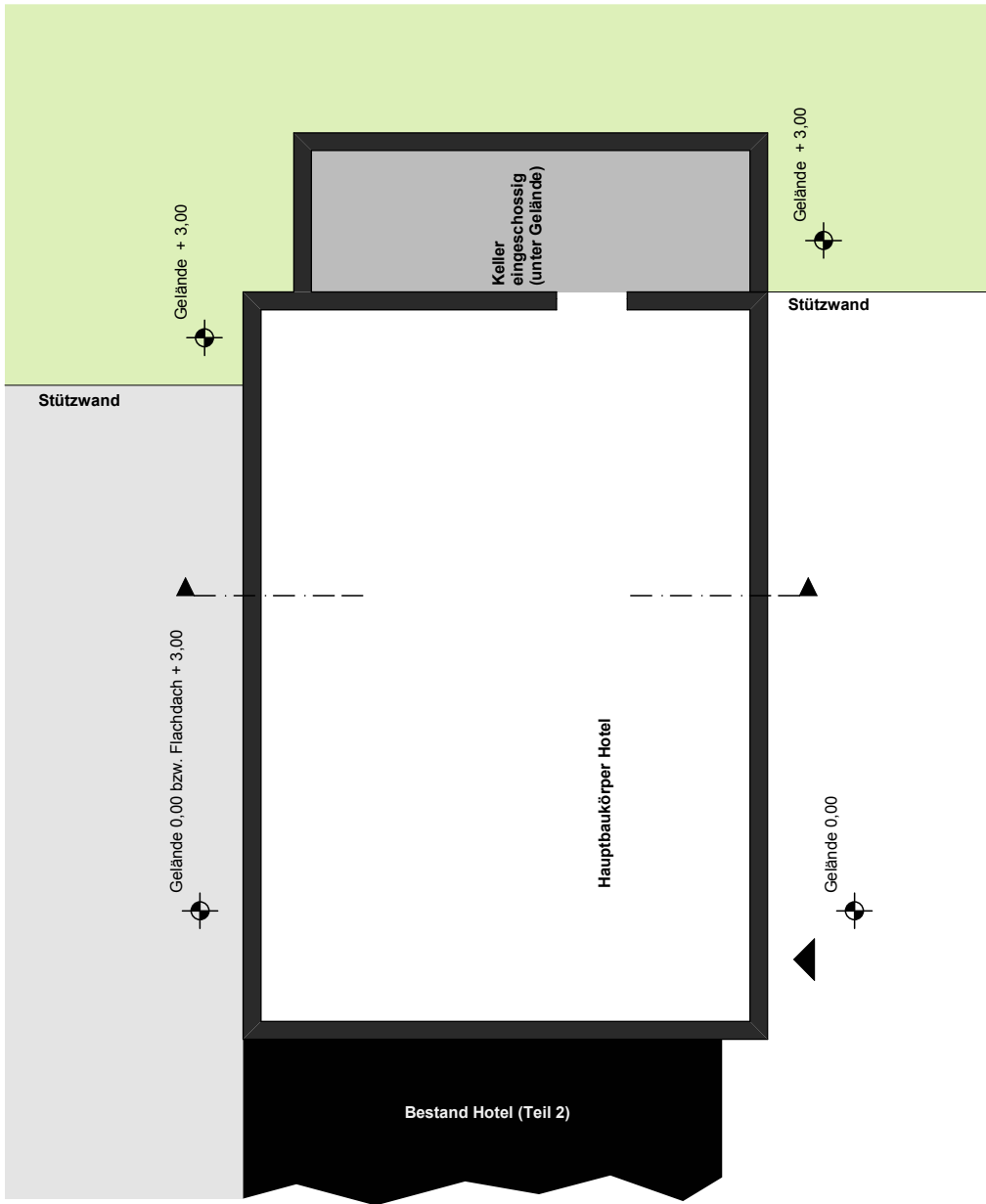
GRUNDRISS (SCHEMATISCH)
