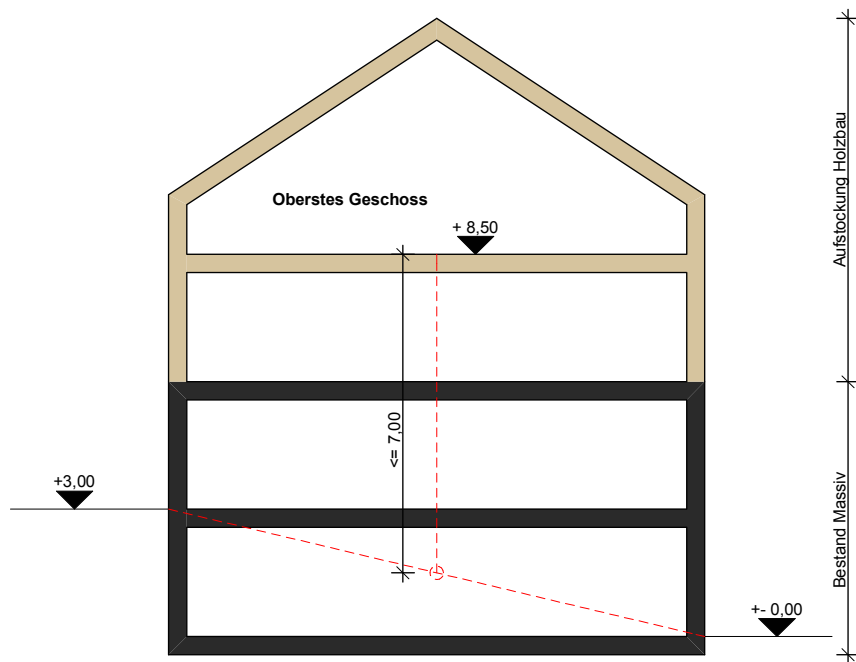
SCHNITT (SCHEMATISCH)
